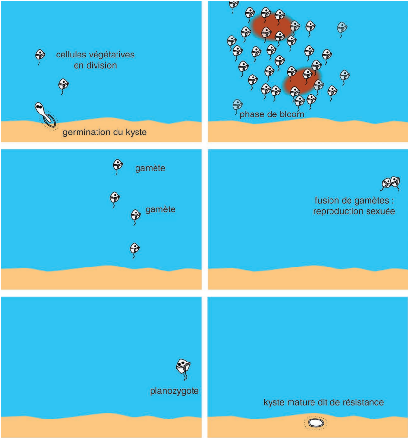
Figure 11. Cycle biologique d' Alexandrium minutum (d'après Wyatt et Jenkinson, 1997). Extrait du site Ifremer environnement littoral.
