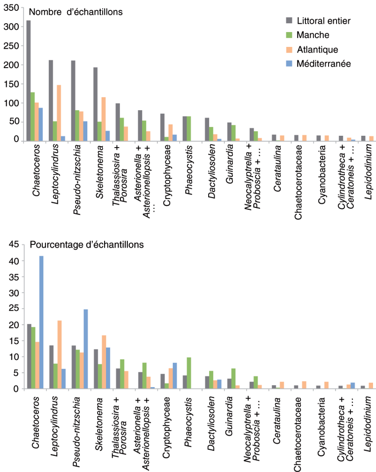
Figure 8. Les seize premières unités taxinomiques ayant contribué à l'indice d'abondance sur la période 2011-2016, pour l'ensemble du littoral français et pour chacune des façades.
