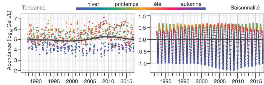
Figure 17. Résultat du modèle linéaire dynamique pour l'abondance phytoplanctonique estimée par la somme des cellules des embranchements Ochrophyta et Myzozoa (incluant les diatomées et dinoflagellés) au lieu de surveillance 063-P-002 Ouest Loscolo, en baie de Vilaine, Bretagne Sud. Explications détaillées voir légende de la figure 15.
