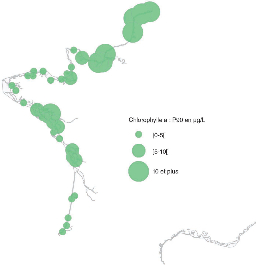
Carte 8. Carte des P90 de chlorophylle a (en µg/L), pour la période 2007-2016 en Manche et Atlantique, sur les masses d'eau affichées dans la figure 23.
